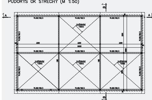
PŮDORYS OK STŘECHY (M 1:50)
