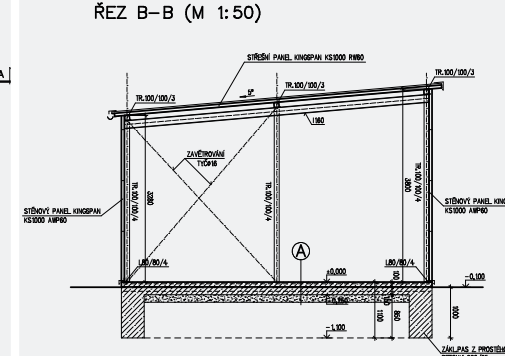
ŘEZ B-B (M 1:50)
