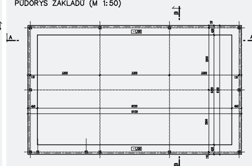
PŮDORYS ZÁKLADŮ (M 1:50)
