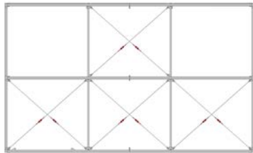
PŮDORYS OK STŘECHY (M 1:50)
