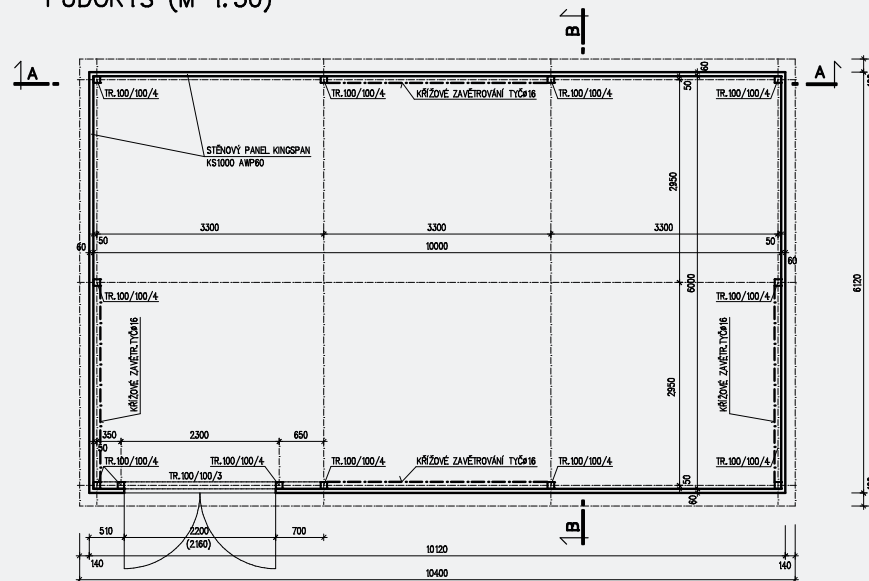
PŮDORYS (M 1:50)
